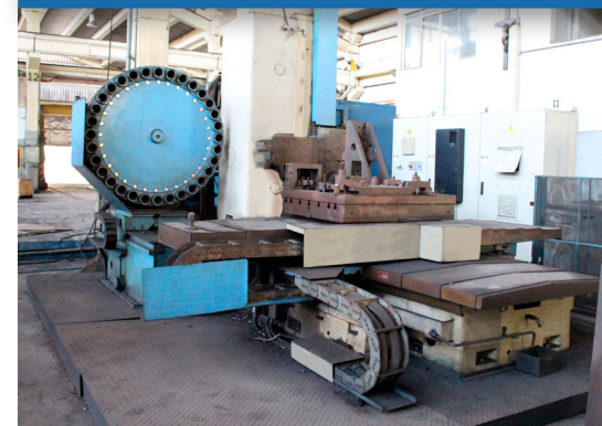
Mandrilhadora com Platô Wotan
