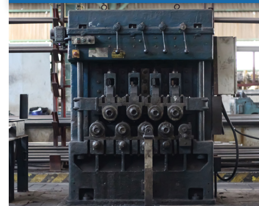
Endiretadora de La- minados Automática
